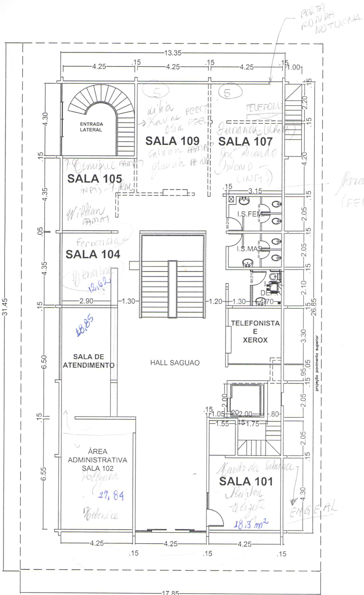
PLANTA BAIXA 1º PAVIMENTO
